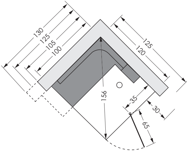
Draufsicht, Abb. Anschlag rechts, Sitz links
